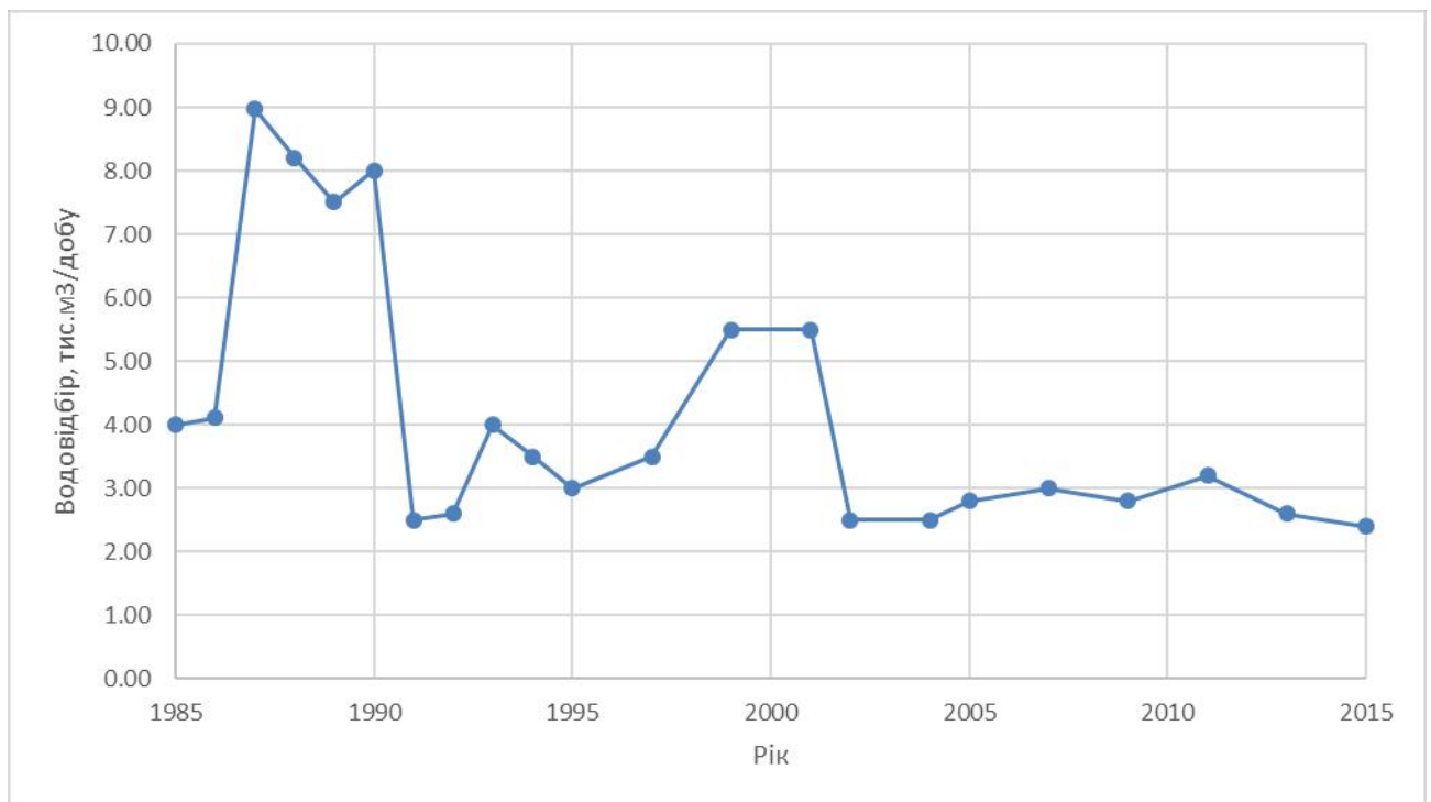
Рис. 3.11. Дані водовідбору на Центральному водозаборі м. Карлівка за 1985-2015 рр. (побудовано автором за звітними матеріалами КП «Південукргеологія»)
