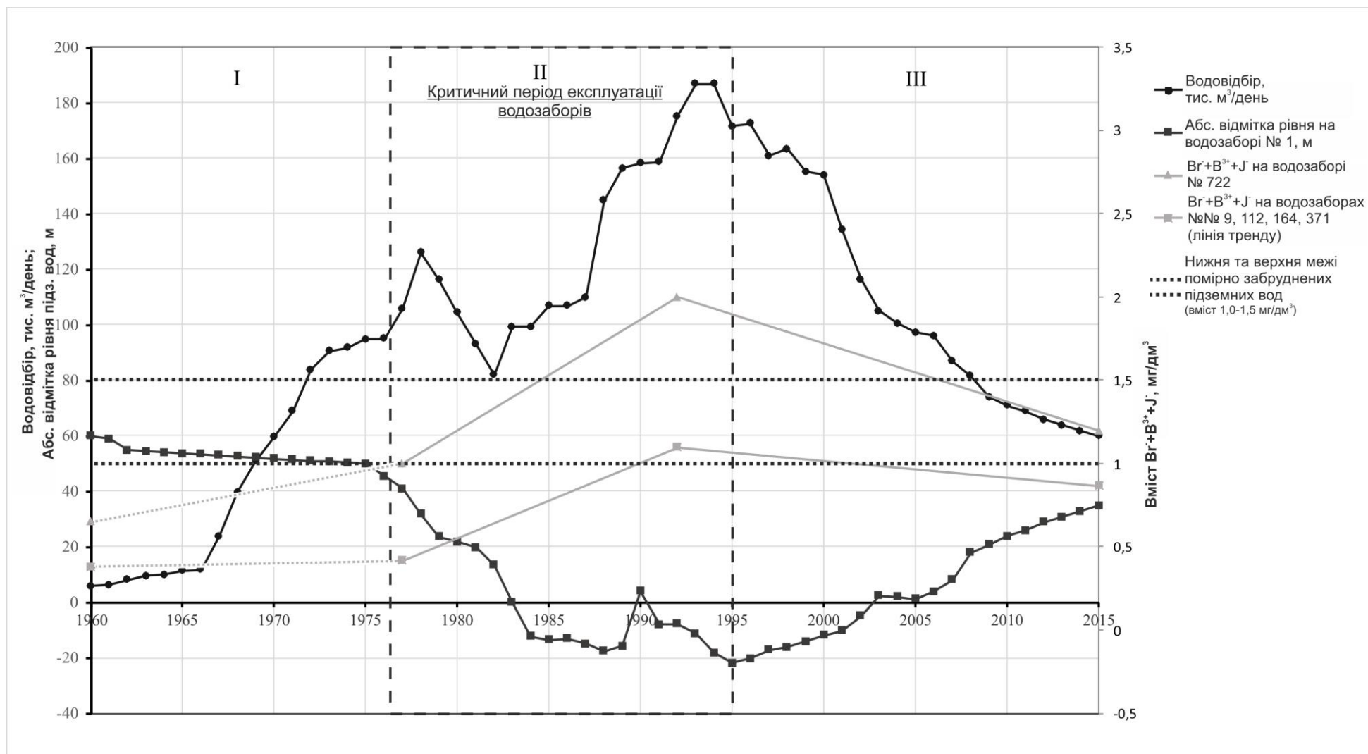
Рис. 5.5. Результати моніторингових досліджень за водовідбором, рівневим режимом та вмістом \text{Br}^- , \text{V}^{3+} , \text{J}^- на водозаборах м. Полтава (побудовано автором)
