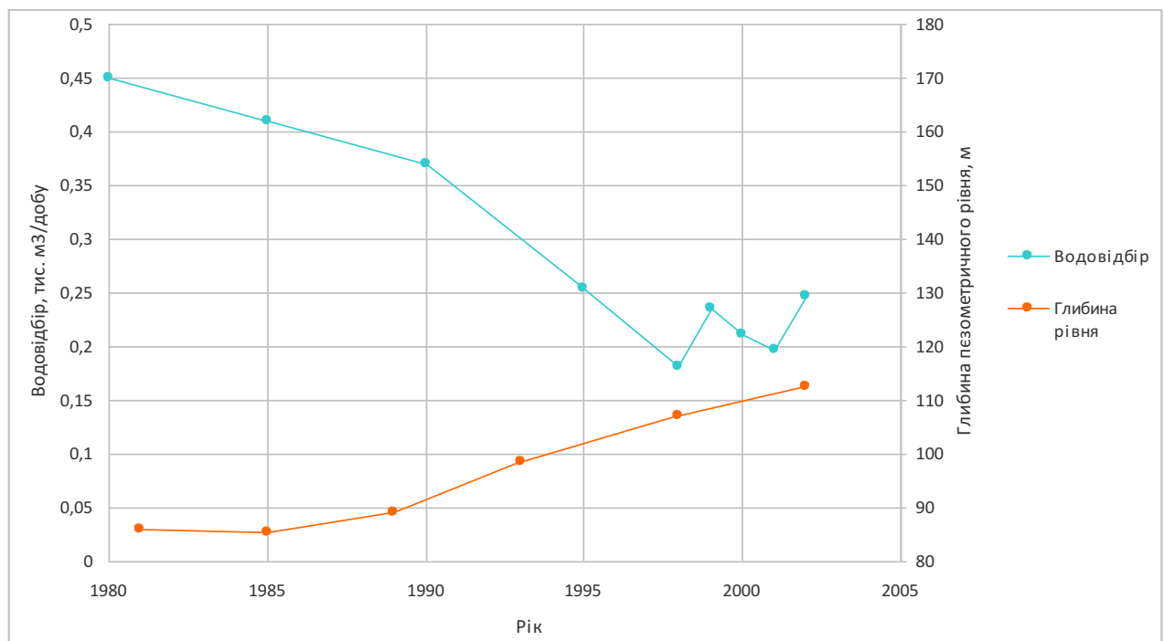
Рис. 3.7. Дані режимних спостережень на водозаборі «Тарапунька» м. Полтава за 1980-2002 рр. (побудовано автором за звітними матеріалами КП «Південукргеологія»)
